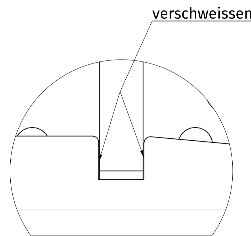
DETAIL X MAßSTAB 2 : 1
